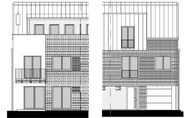
ZAHRADNÍ POHLED
